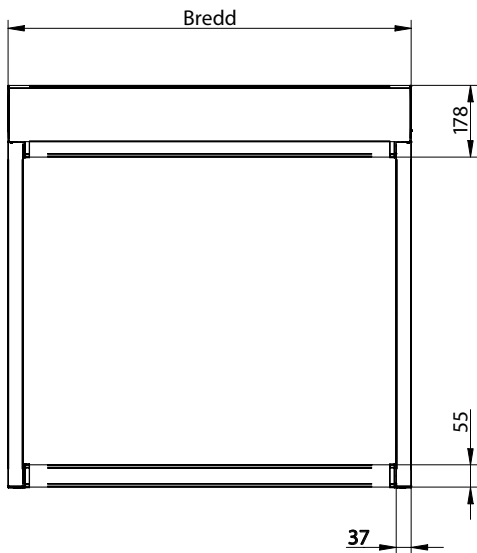
Frontvy 4K
