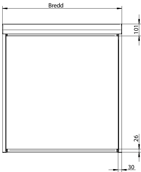
Frontvy
