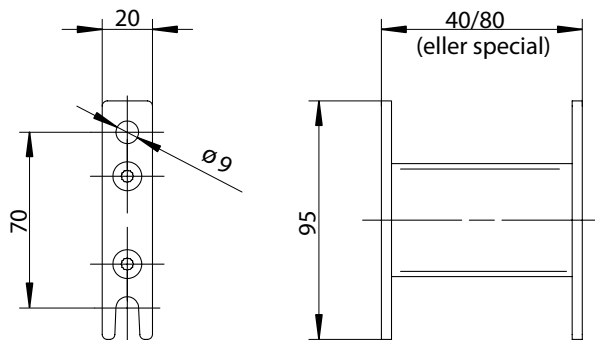
Avståndshållare (tillval)
