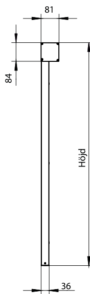
Sidovy 4K
