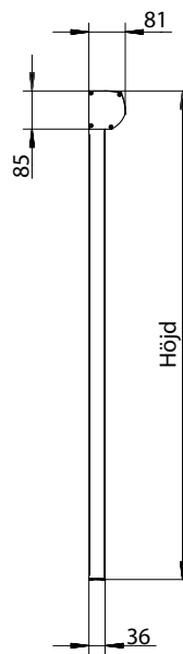
Sidovy
