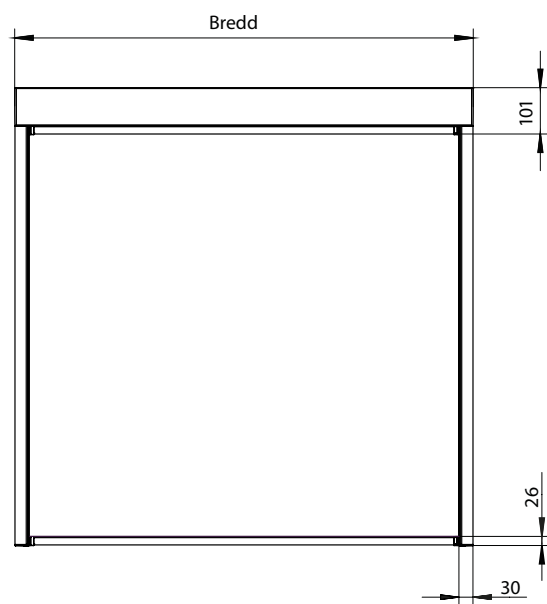
Frontvy 4K
