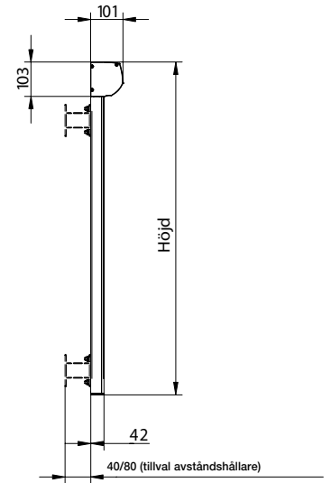
Snäppskena
