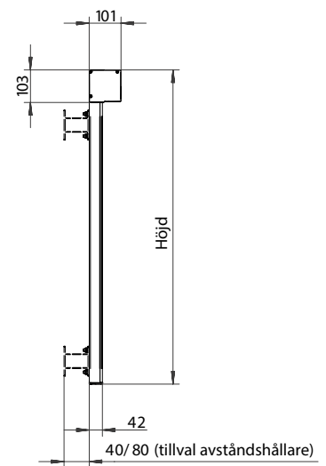
Snäppskena
