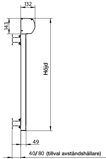
Sidovy
