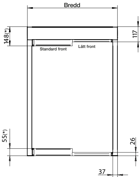
Frontvy 4K
