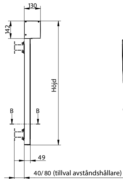
Sidovy 4K
